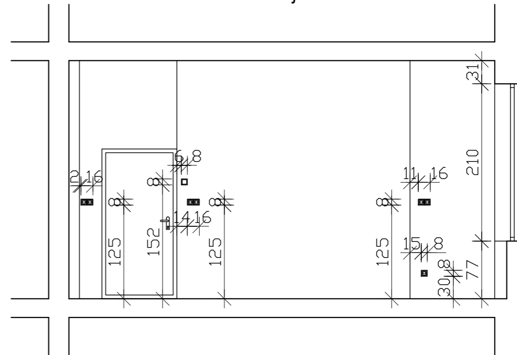
Przekrój D-D
