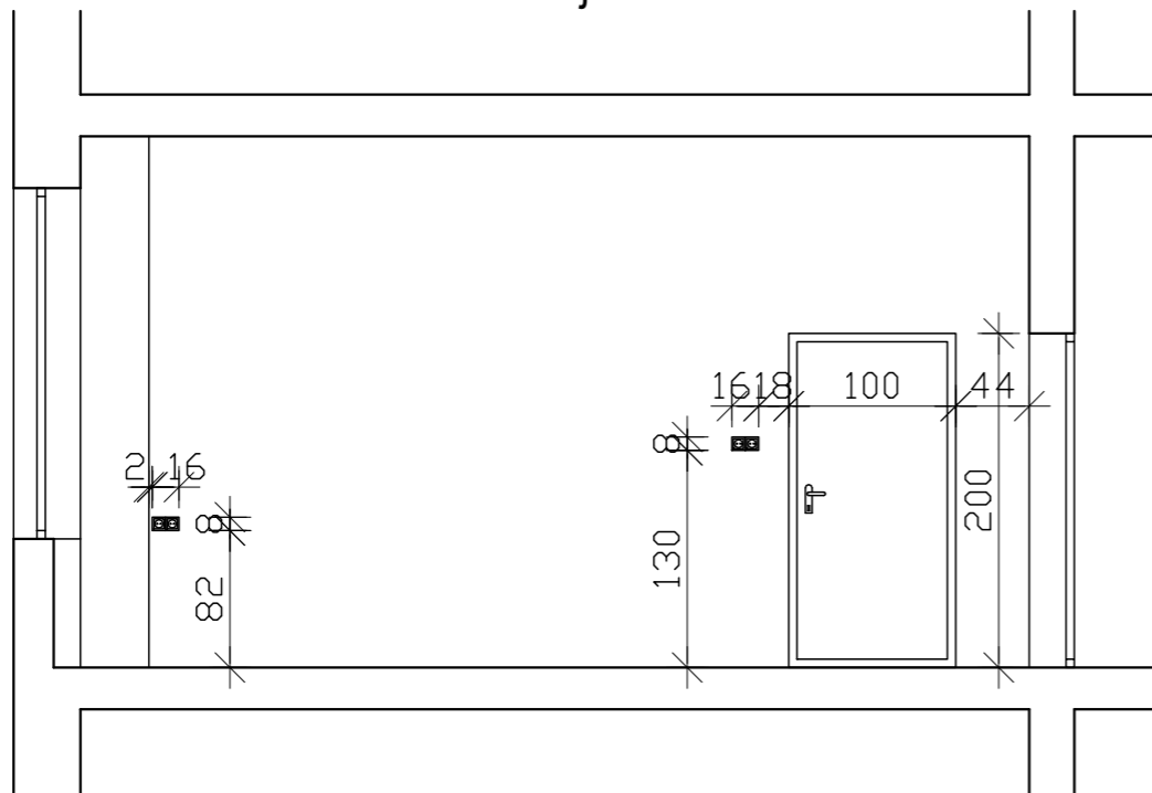
Przekrój E-E
